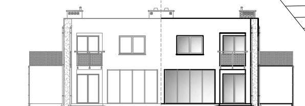
ELEVACJA OGRODOWA
